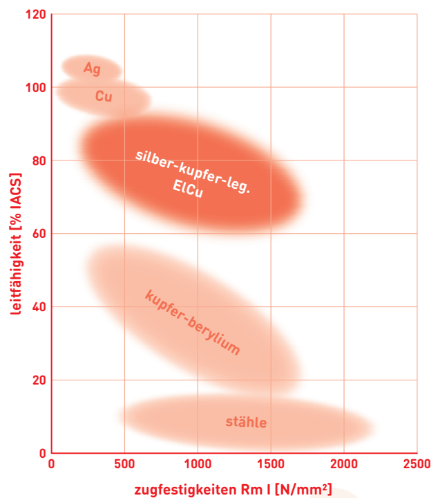
grafische einordnung gebräuchlicher materialien nach elektrischer leitfähigkeit und zugfestigkeit
